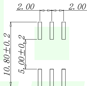
印制线路板 PCB Layout Recommended
