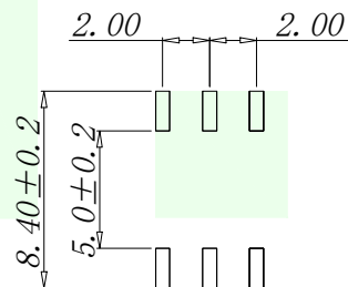
印制线路板 PCB Layout Recommended
