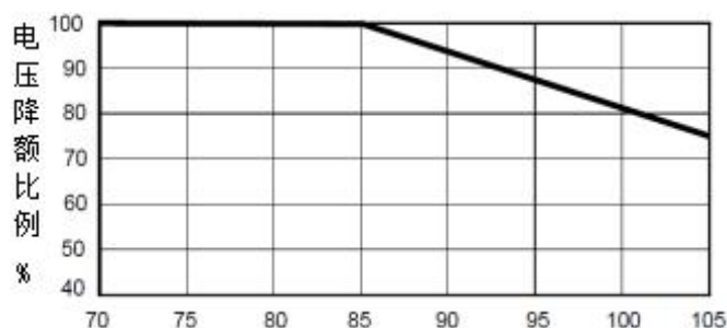
额定电压降额曲线
