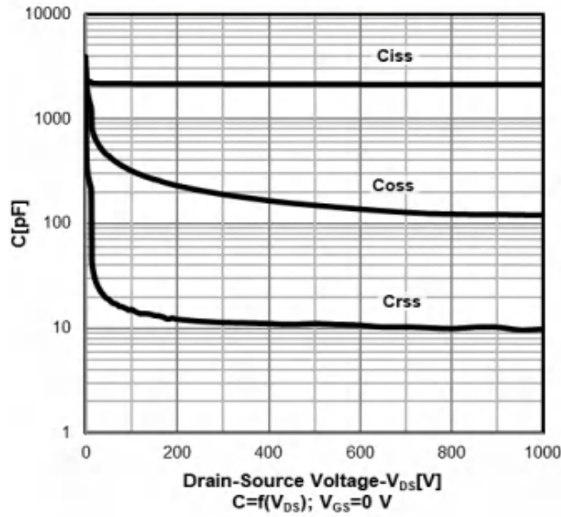
Typ. capacitances
