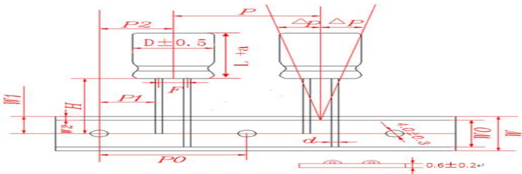
Φ10-Φ12.5
