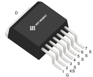
TO-263-7L
