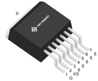
TO-263-7L
