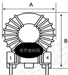
正视图 front view
