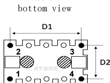
底视图 bottom view
