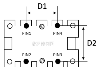
底视图 bottom view
