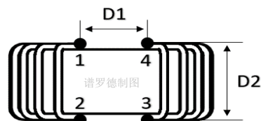
底视图 Bottom view
