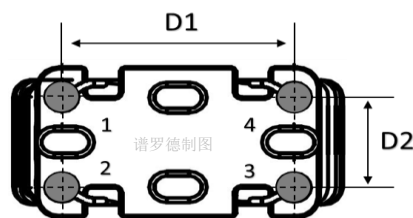
底视图 bottom view
