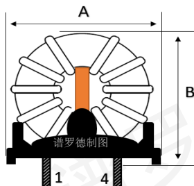
正视图 front view
