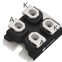
SOT-227
