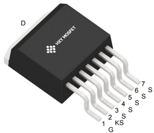
TO-263-7L
