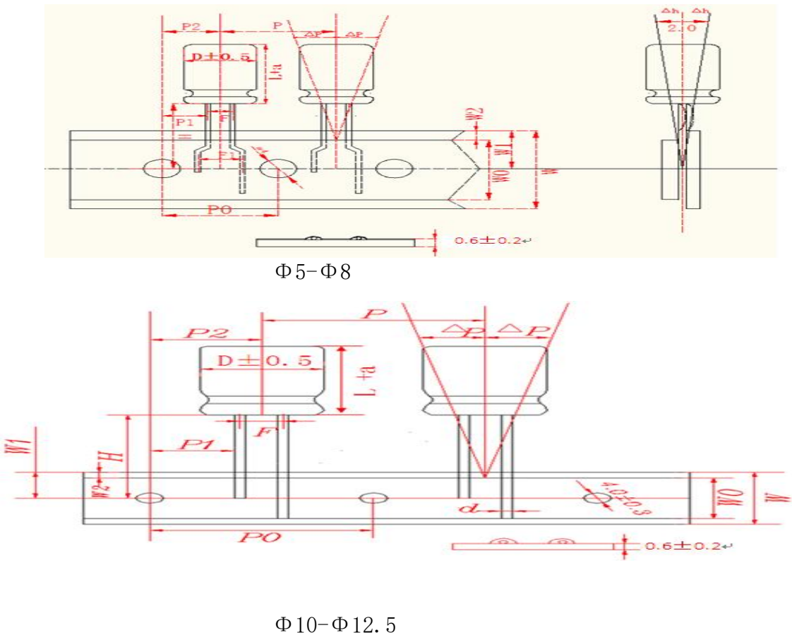
编带外型尺寸 B 图
