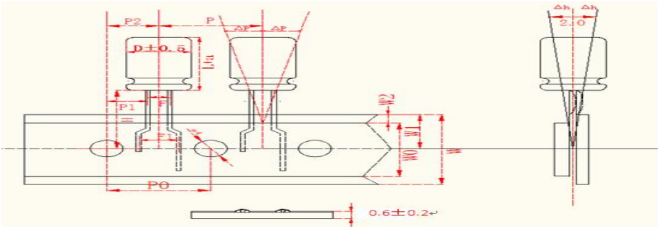
编带外型尺寸 B 图
