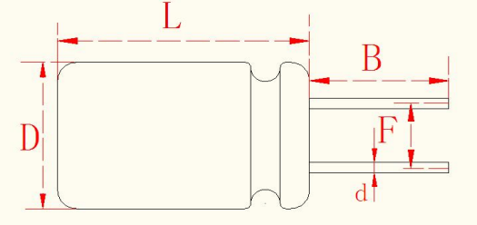
引线切脚成型 B 图
