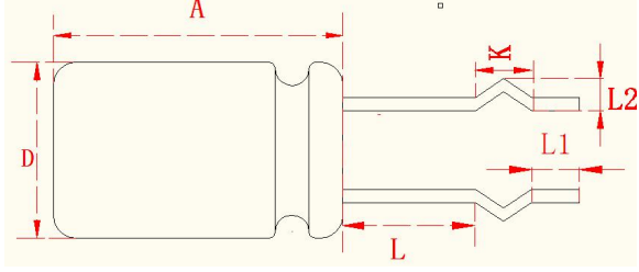
引线切脚成型 C 图
