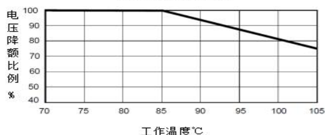
额定电压降额曲线
