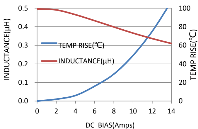
VCMA-0420-R47-M-1A
