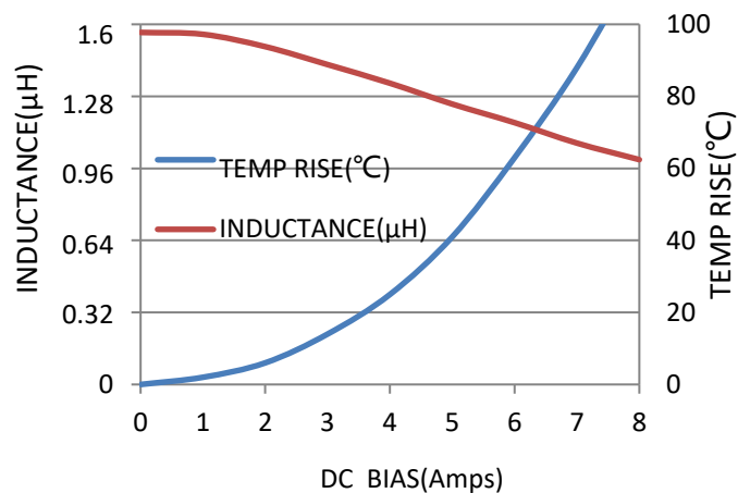
VCMA-0420-1R5-M-1A
