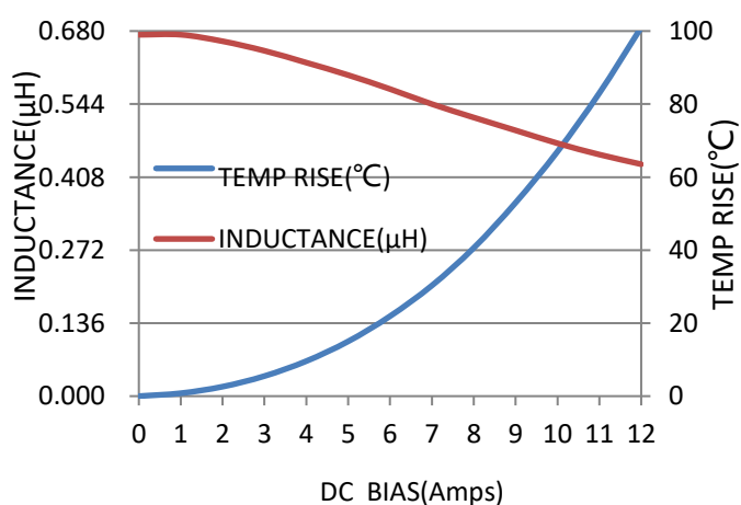
VCMA-0420-R68-M-1A
