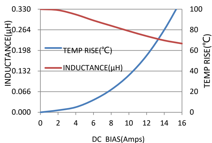
VCMA-0420-R33-M-1A
