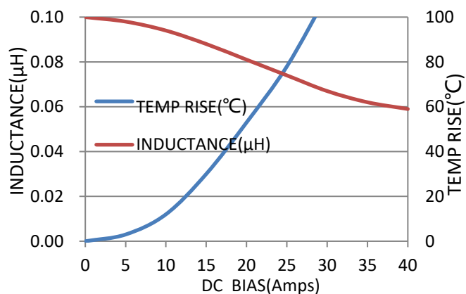
VCMA-0420-R10-M-1A
