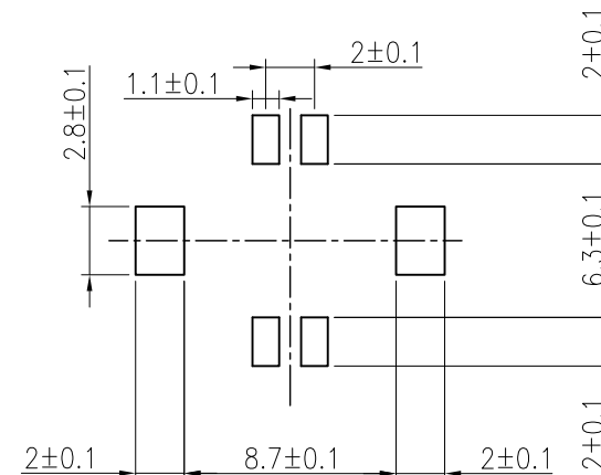
P.C.B LAYOUT
