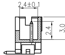
SEC:A-A
