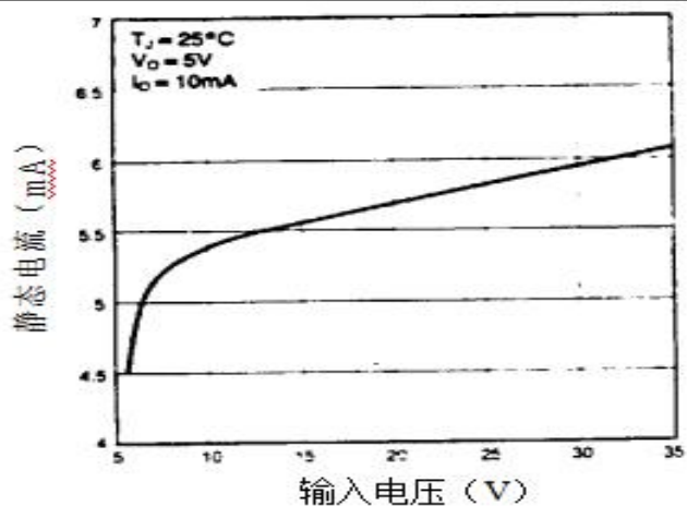
静态电流
