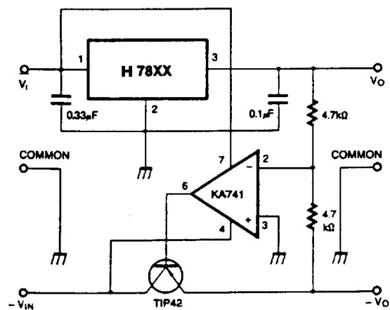
图 10、跟踪稳压器
