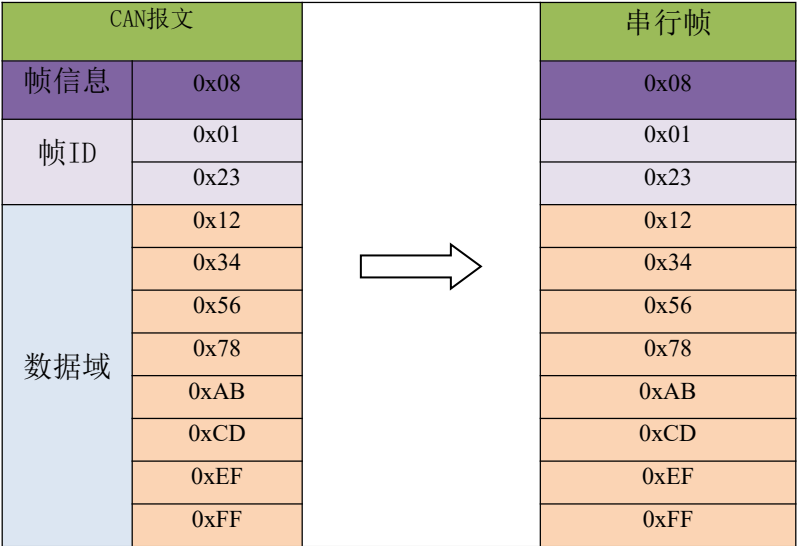
CAN报文转换成串行帧 （透明方式）
