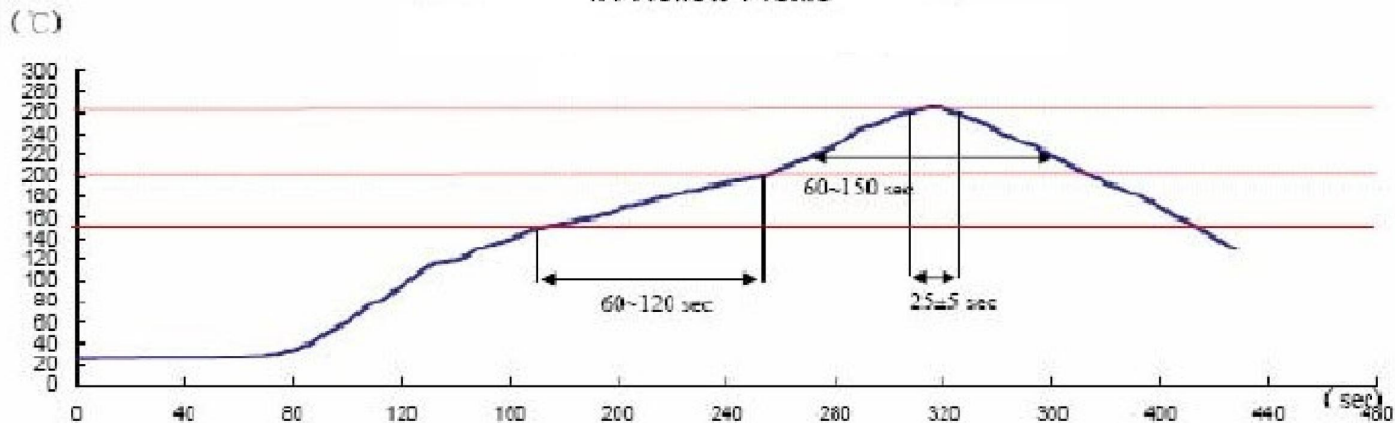
IR-Reflow Profile
