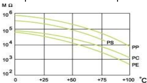
绝缘电阻与温度的关系
