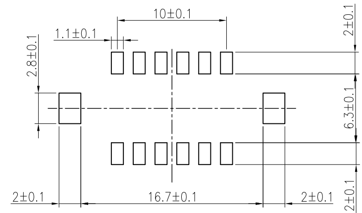
P.C.B LAYOUT
