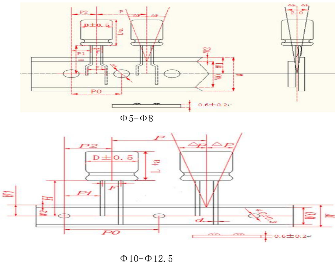
编带外型尺寸 B 图
