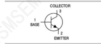
SOT-89
