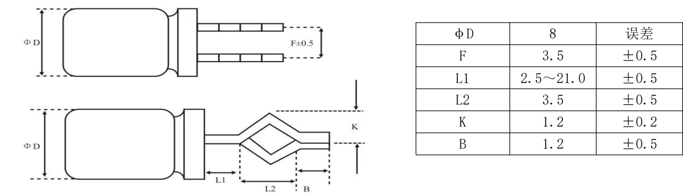
引线切脚成型 D 图
