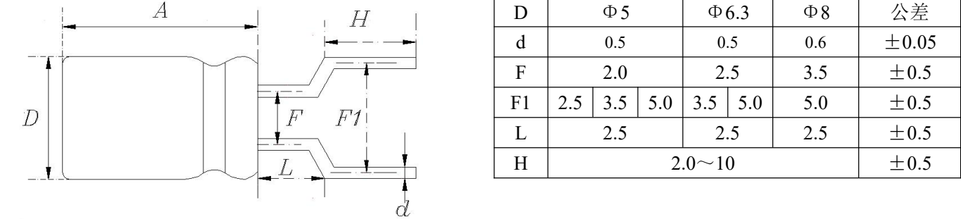
引线切脚成型 G 图
