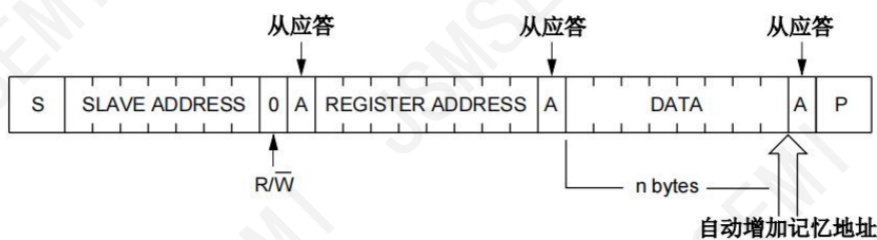
图 11 主传送器到从接收器（写模式）
