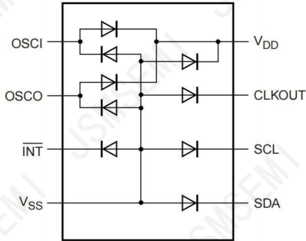
图2 内部二极管保护框图
