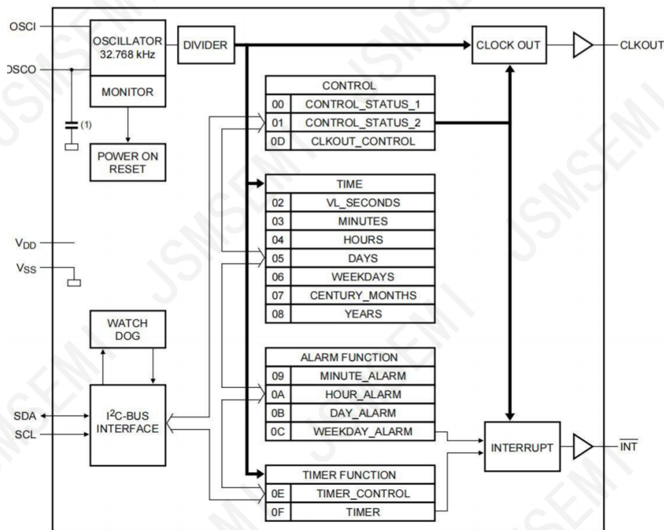
图1 内部功能框图
