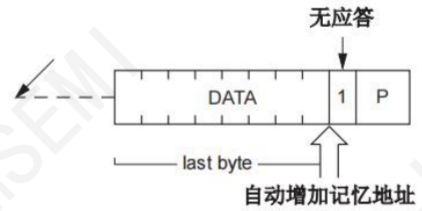
图 12 设置字节地址后主设备读数据（写字地址：读数据）
