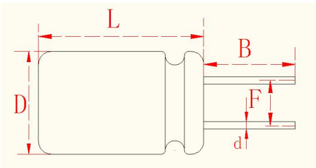
引线切脚 A 图
