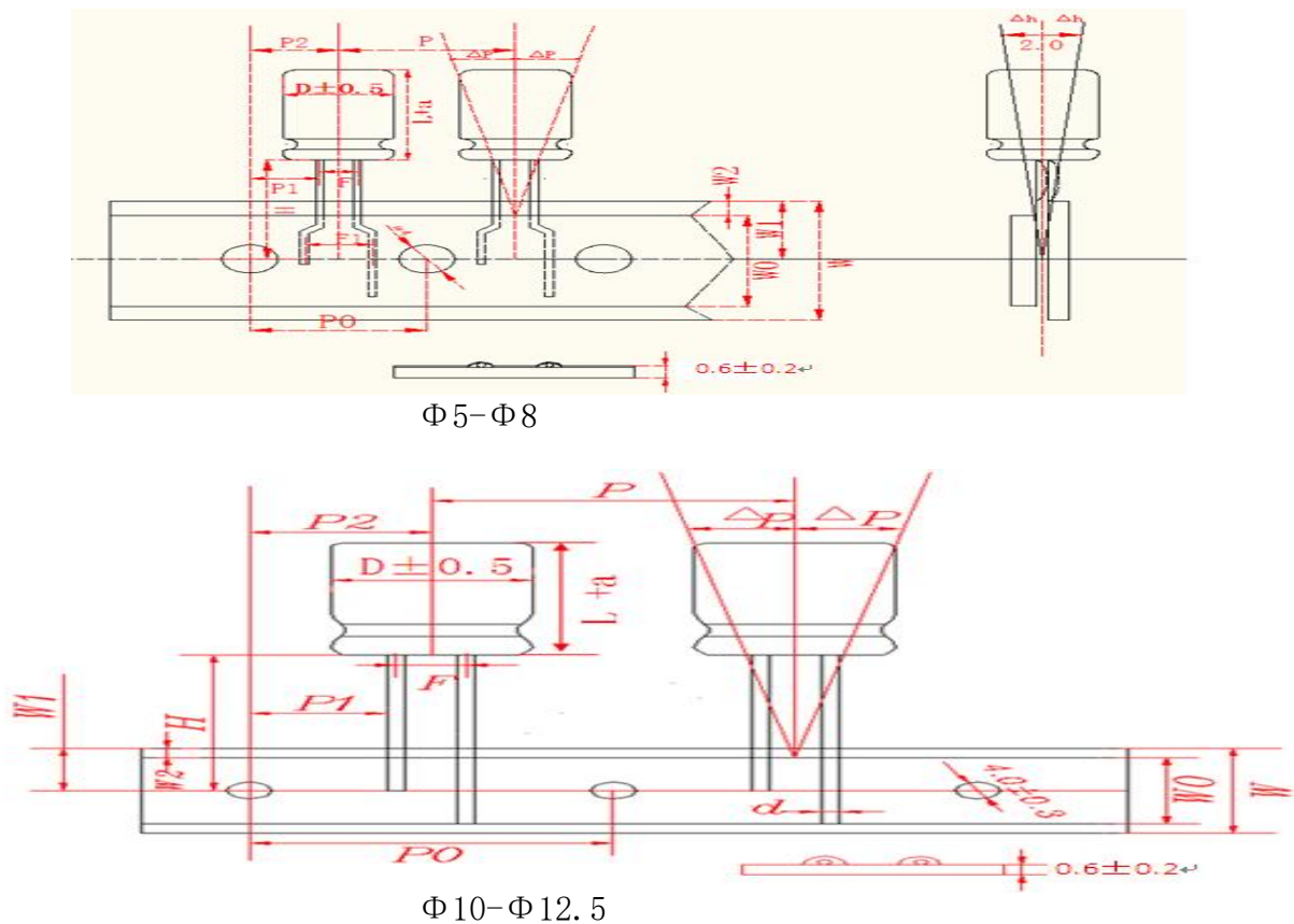
编带外型尺寸 B 图
