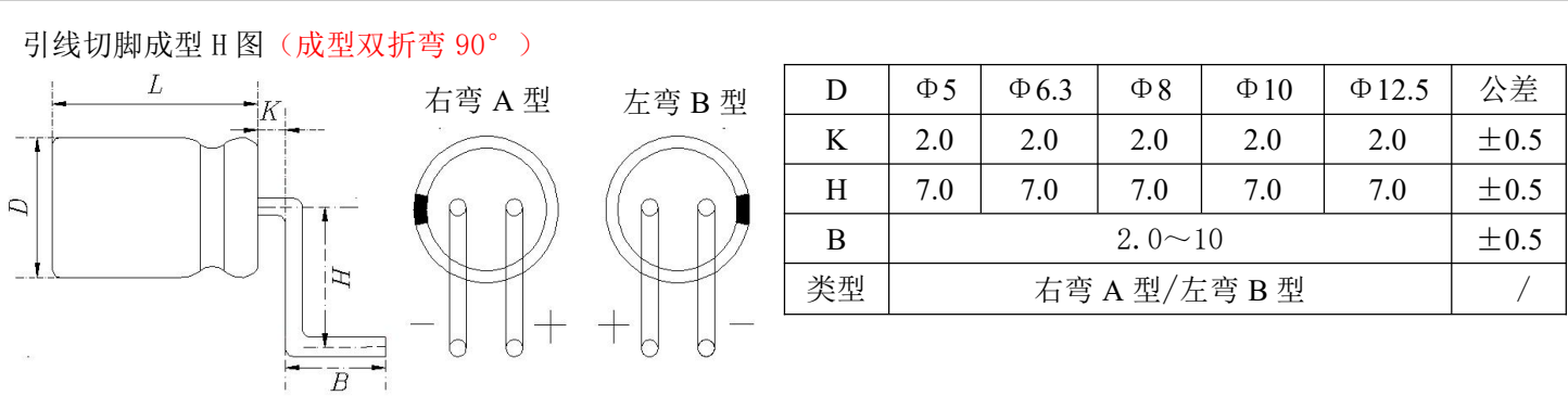
编带外型尺寸 A 图
