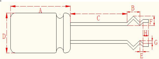
引线切脚成型 C 图
