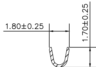
SEC:B-B
