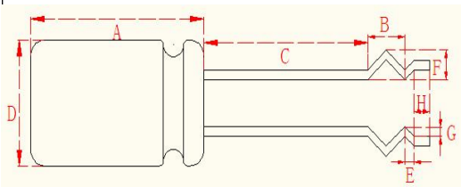
引线切脚成型 C 图
