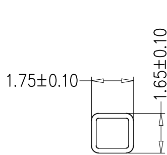
SEC: D-D
