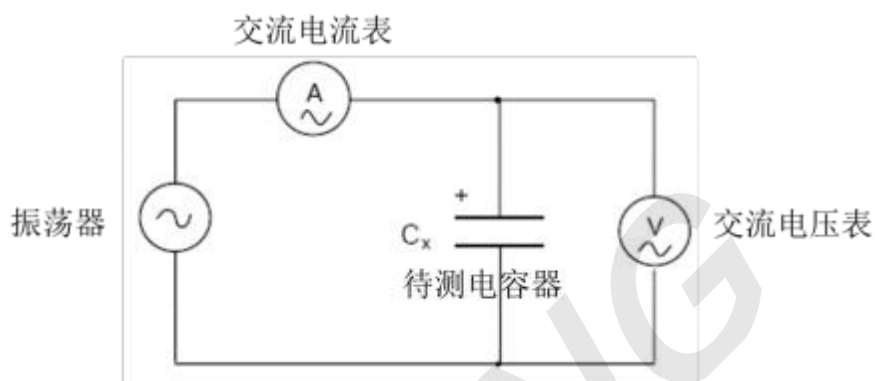
图3 交流阻抗电路
