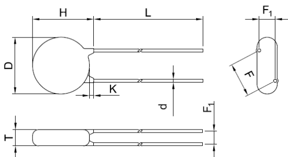
仰视图 Bottom View
