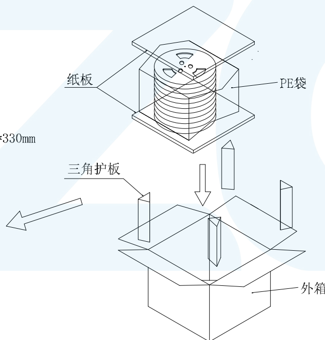
④ 产品入外箱示意图
