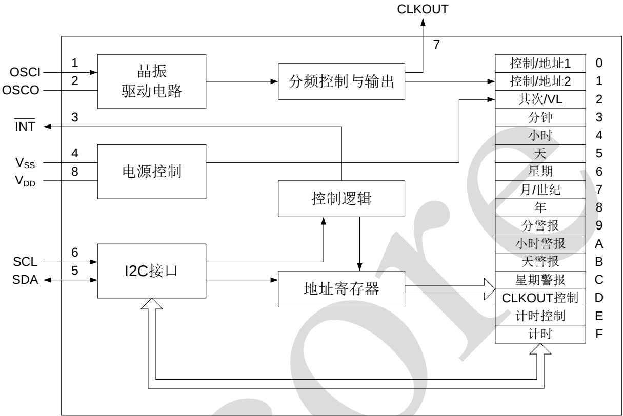
图 1、功能框图
