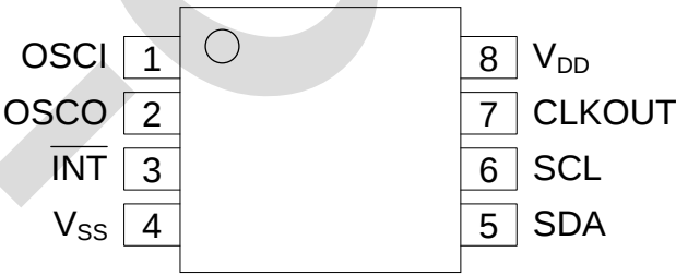
图 2、引脚图
