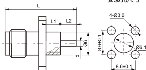
安装孔尺寸
