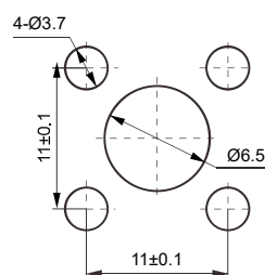
安装孔尺寸
