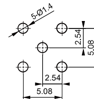
安装孔尺寸
