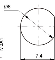
安装孔尺寸
