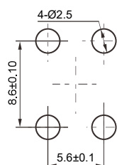
安装孔尺寸
