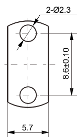
法兰盘尺寸
