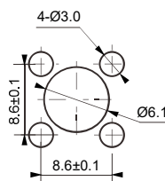
安装孔尺寸
