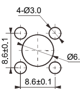
安装孔尺寸
