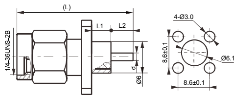
安装孔尺寸
