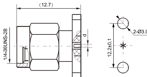
安装孔尺寸
