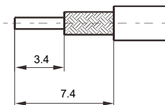
电缆剥线尺寸
