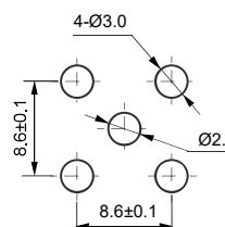
安装孔尺寸
