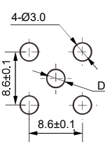
安装孔尺寸
