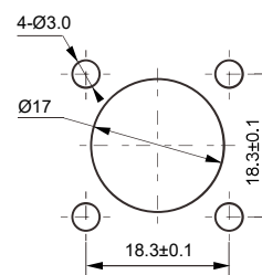
安装孔尺寸
