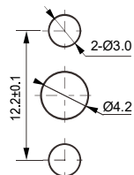
安装孔尺寸
