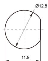
安装孔尺寸
