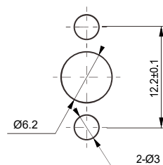
安装孔尺寸
