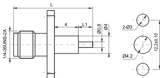
安装孔尺寸
