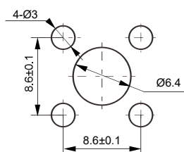
安装孔尺寸
