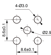
安装孔尺寸
