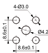
安装孔尺寸
