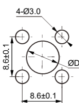
安装孔尺寸
