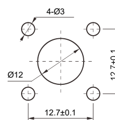
安装孔尺寸
