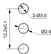
安装孔尺寸
