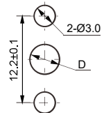
安装孔尺寸
