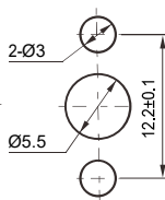
安装孔尺寸
