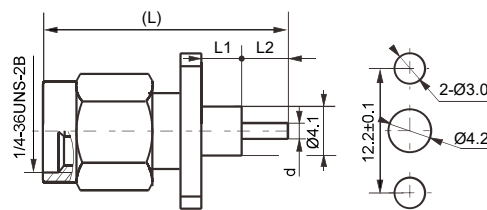
安装孔尺寸
