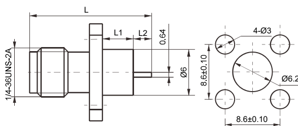
安装孔尺寸
