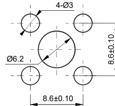
安装孔尺寸
