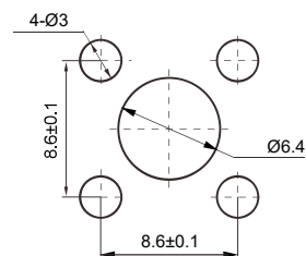
安装孔尺寸
