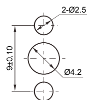
安装孔尺寸
