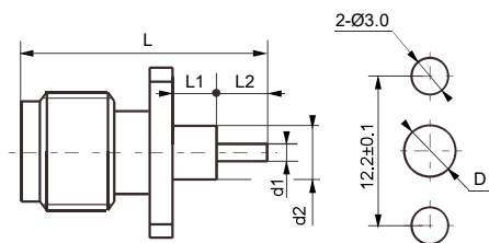
安装孔尺寸
