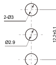
安装孔尺寸
