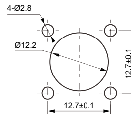
安装孔尺寸
