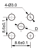
安装孔尺寸
