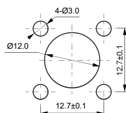
安装孔尺寸
