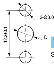
安装孔尺寸
