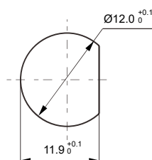
安装孔尺寸
