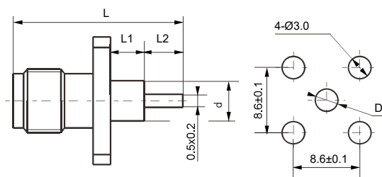
安装孔尺寸
