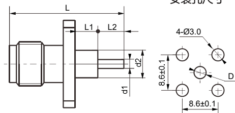
安装孔尺寸
