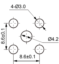
安装孔尺寸
