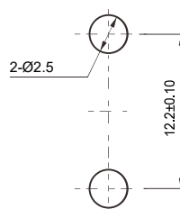
安装孔尺寸
