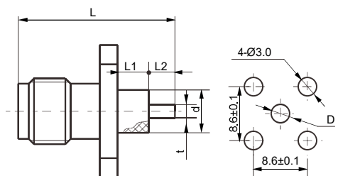
安装孔尺寸
