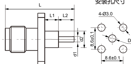
安装孔尺寸
