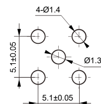
安装孔尺寸
