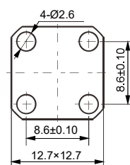
法兰盘尺寸
