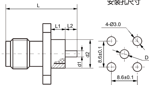
安装孔尺寸
