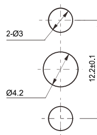
安装孔尺寸
