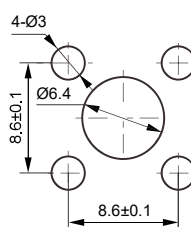
安装孔尺寸
