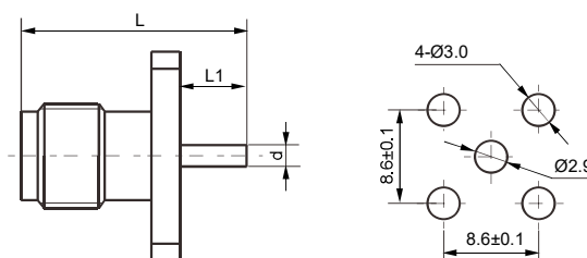
安装孔尺寸
