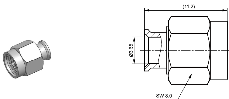
SMA-JB3
