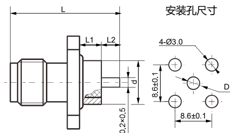
安装孔尺寸
