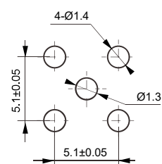
安装孔尺寸
