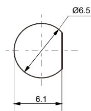
安装孔尺寸
