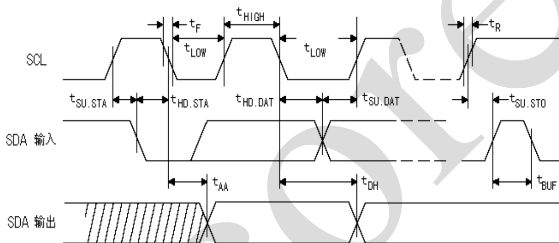
图 5、总线时序
