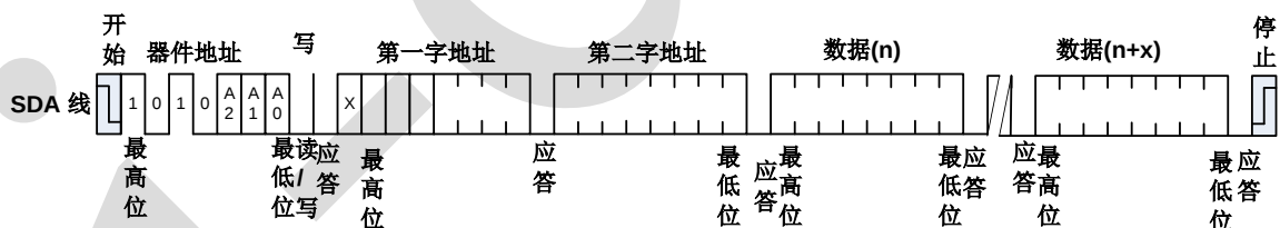
图 9、页写
