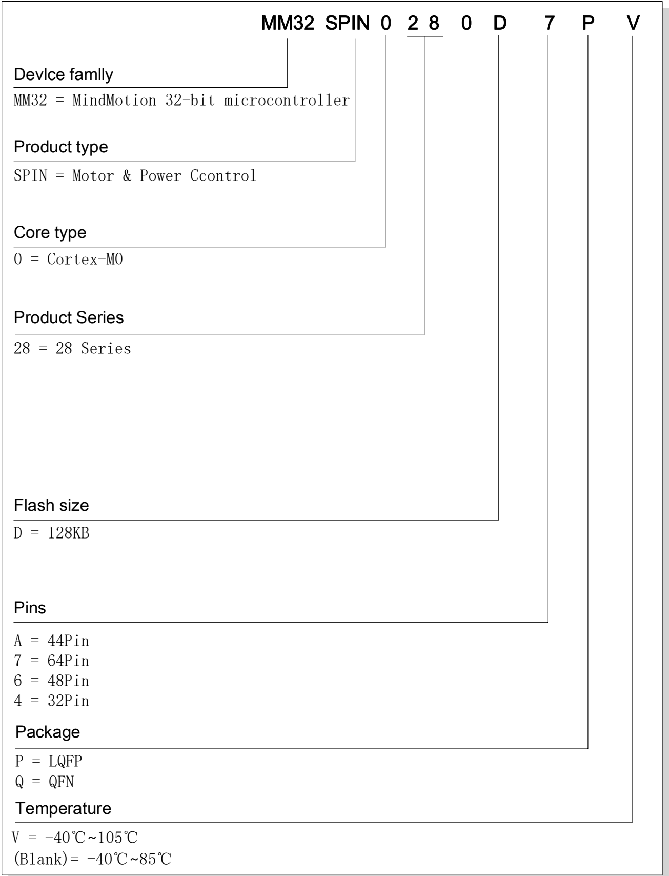
图 21 MM32 型号命名
