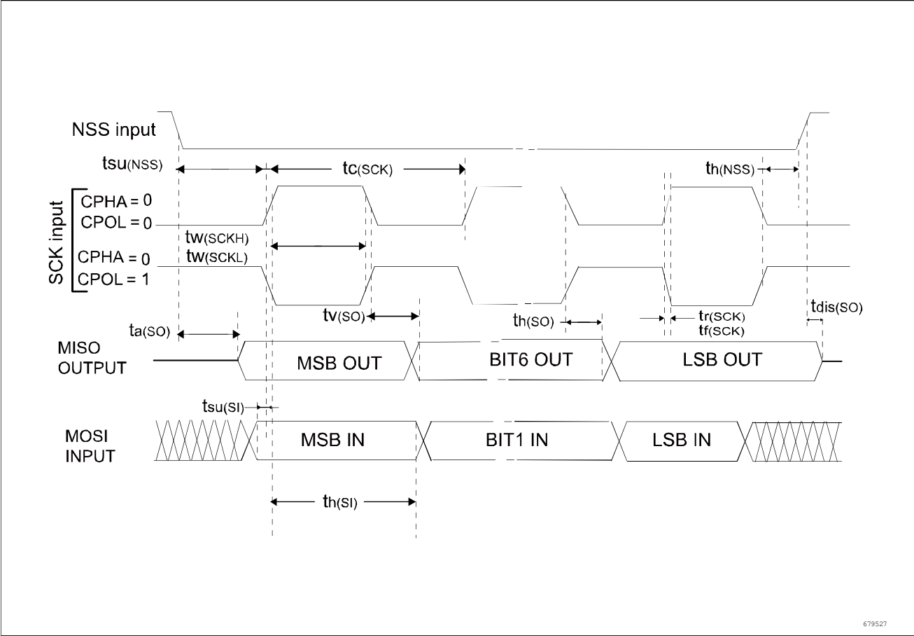
图 15 SPI 时序图-从模式和 CPHA = 0, CPOLSEL = 1
