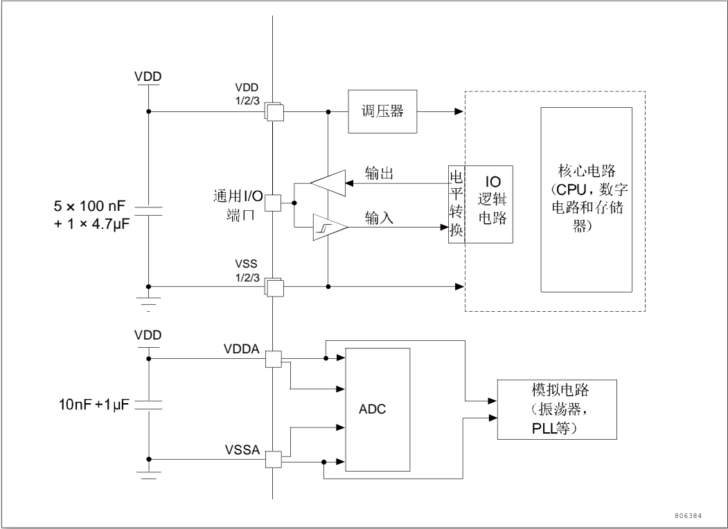
图 7 供电方案
