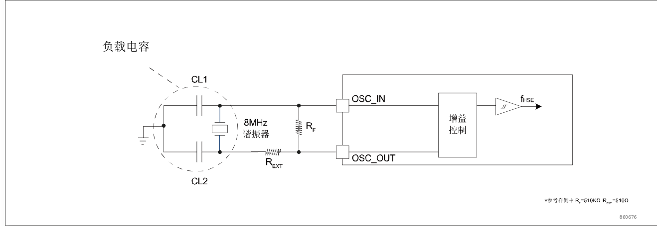
图 11 使用 8MHz 晶体的典型应用
