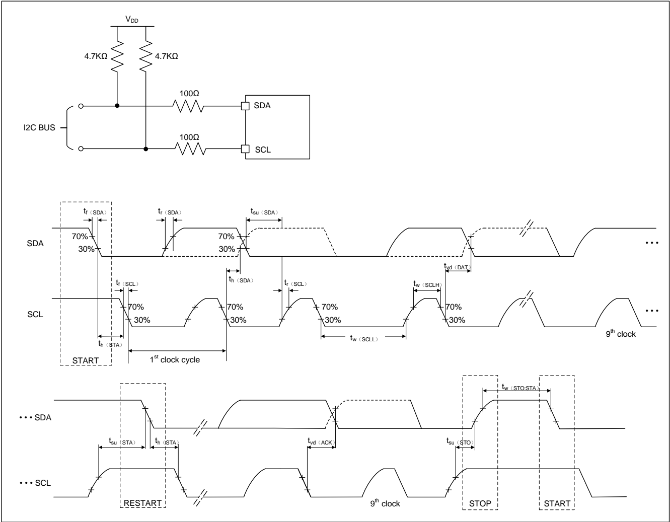
图 14 I2C 总线交流波形和测量电路 (1)
