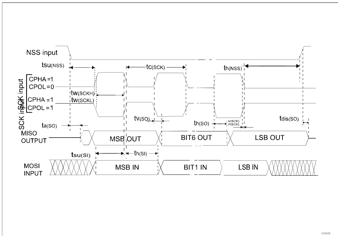
图 16 SPI 时序图-从模式和 CPHA = 1, CPHASEL = 1 (1)
