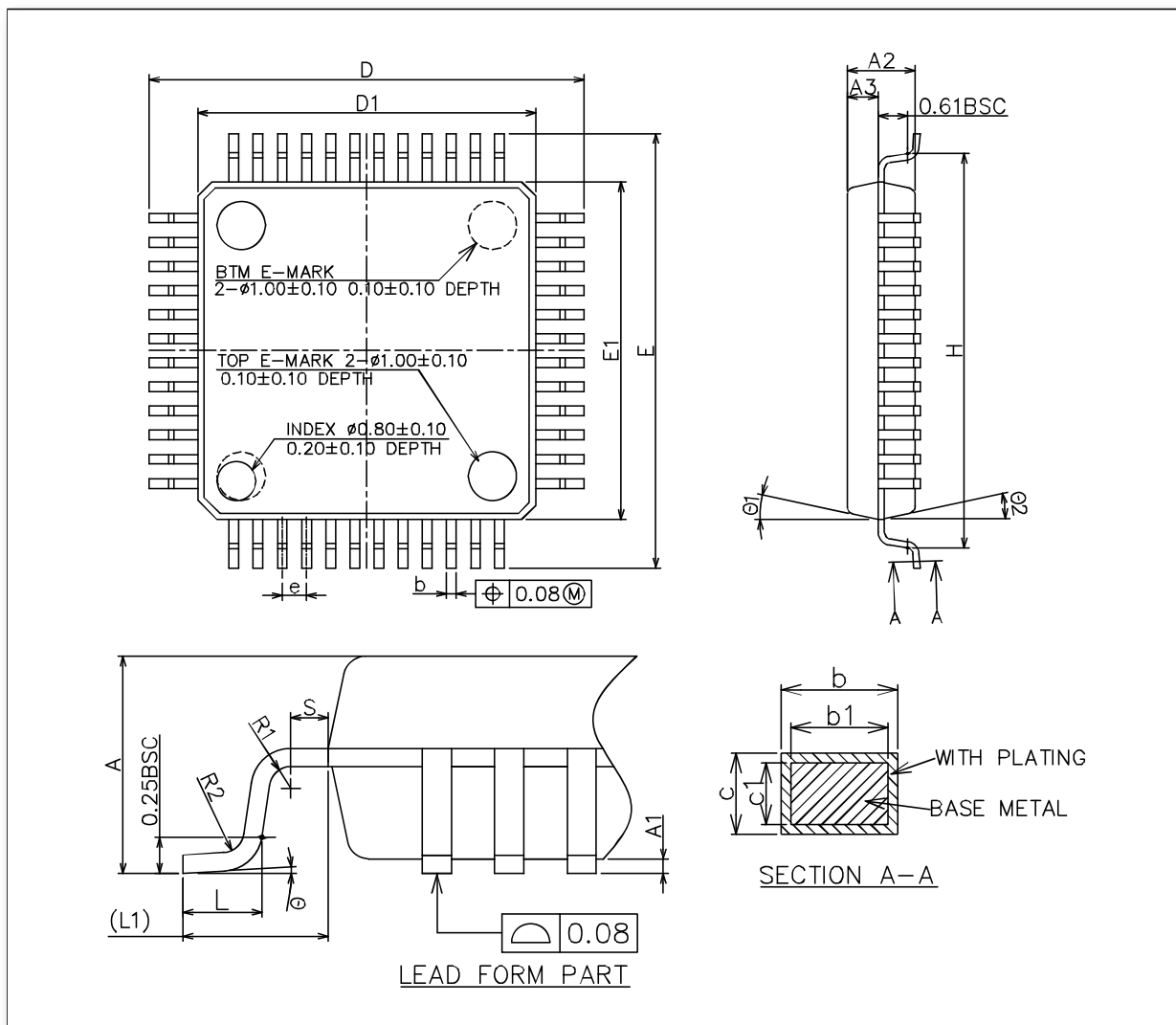
图 20 LQFP48, 48 脚低剖面方形扁平封装图
