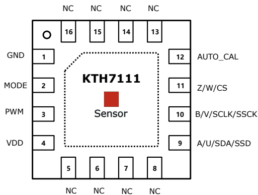
图 3: QFN-16L 3mmx3mm 传感器位于几何中心
