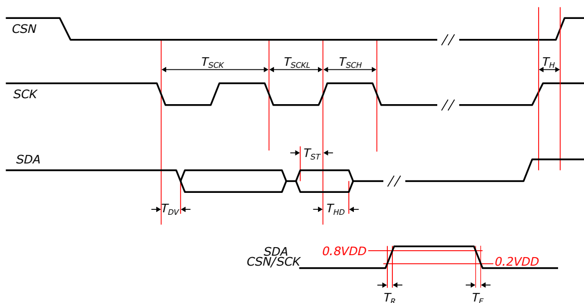
图 6: SPI 时序图
