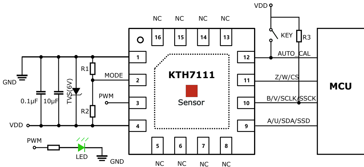
图 2: 应用电路
