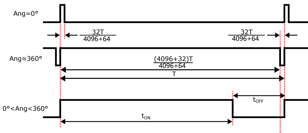
图 18: PWM 时序
