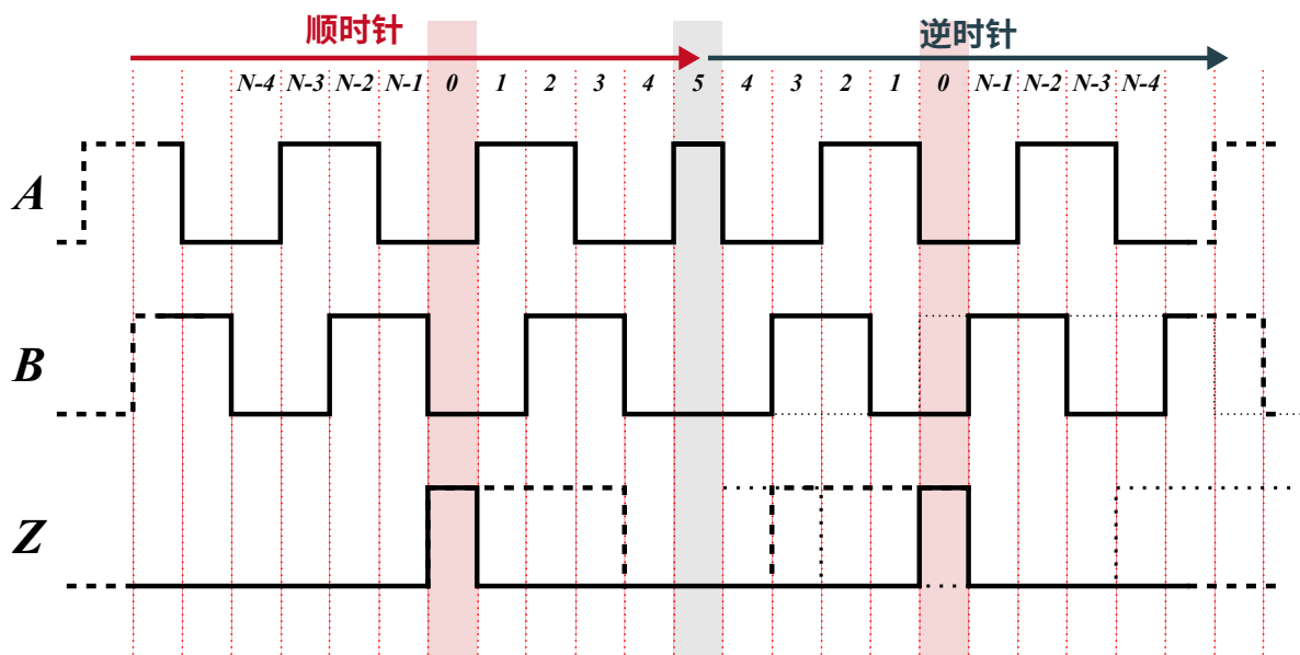
图 15: ABZ 输出时序
