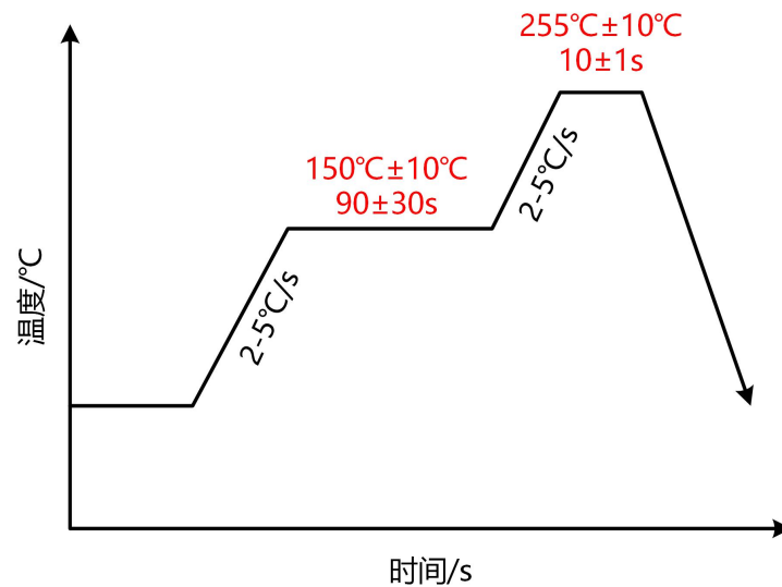
图 23: 焊接温度曲线
