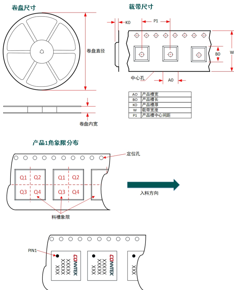
图 22: QFN-16L 卷盘载带尺寸
