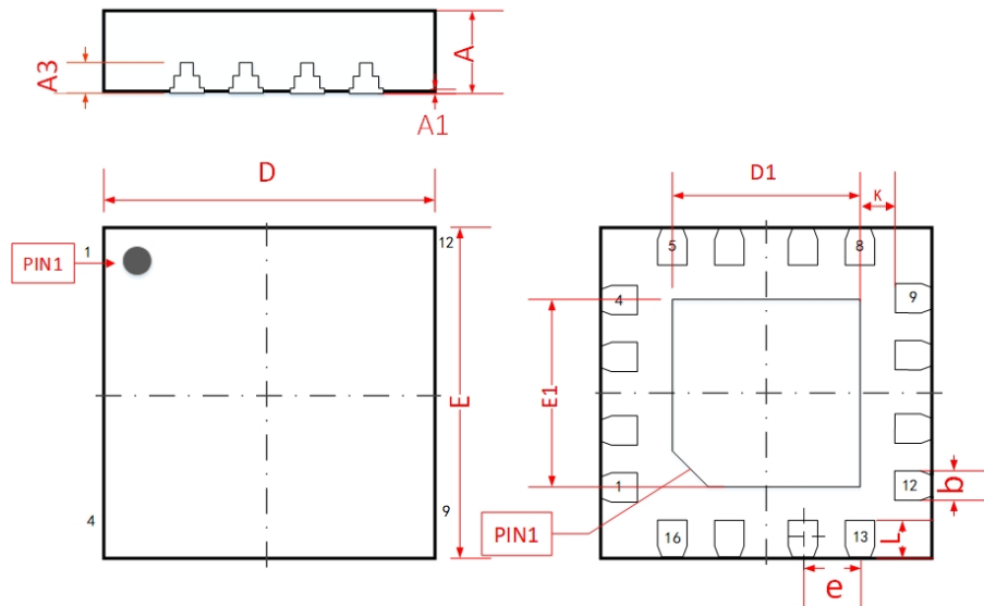
图 21: QFN-16L 封装信息
