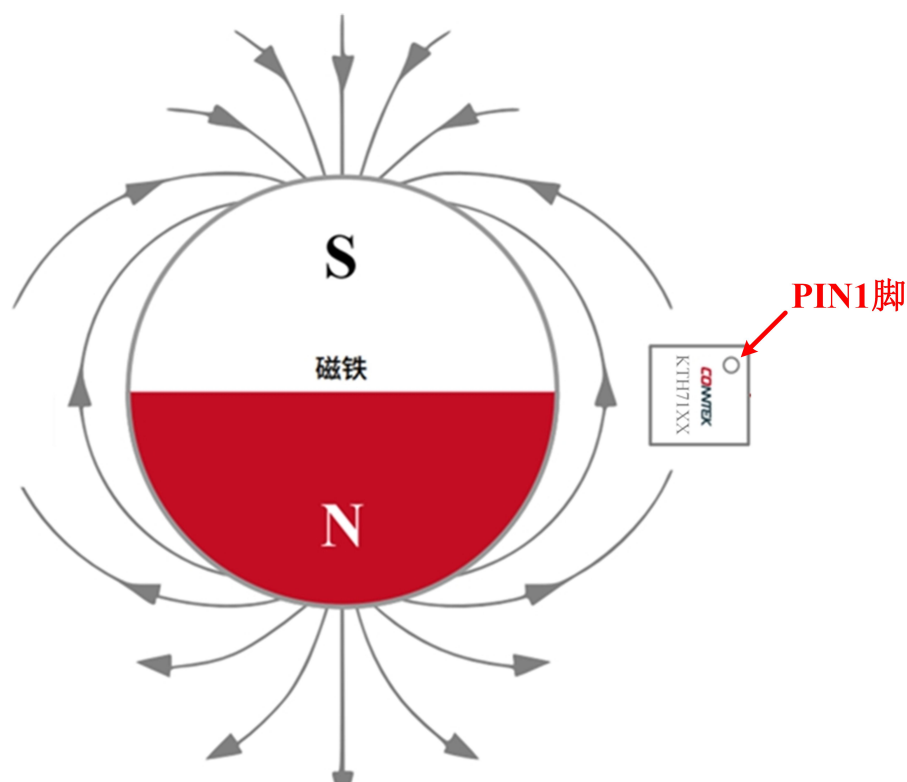
图 19: 芯片摆放方向与磁铁位置示意图
