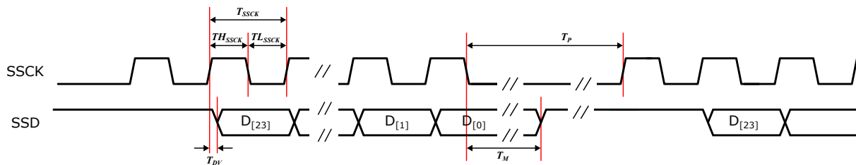
图 13: SSI 接口时序图
