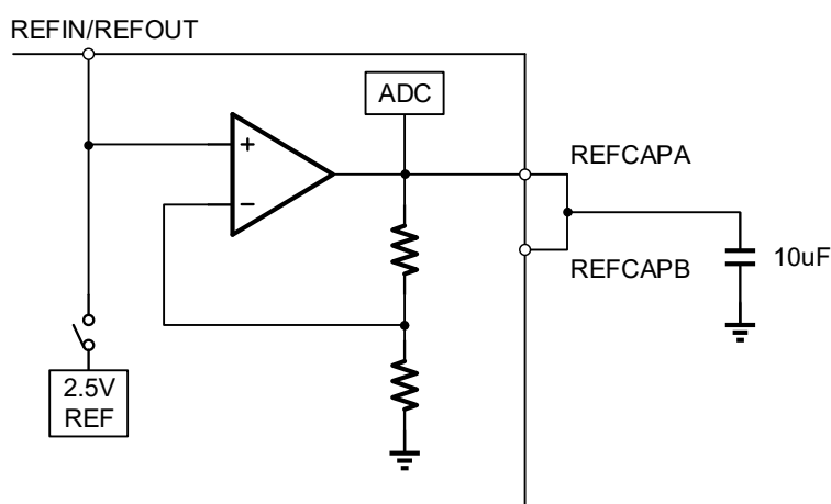
图 12 基准电压电路
