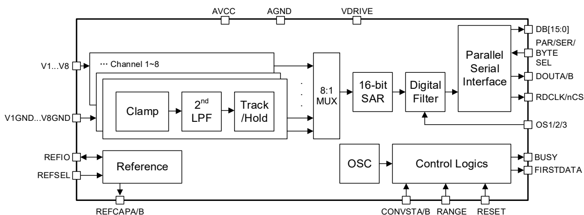
图 1 HT7606 功能框图
