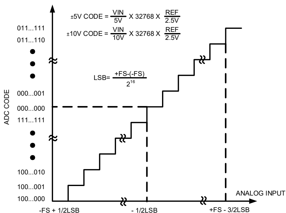
图 11 HT7606 传递函数
