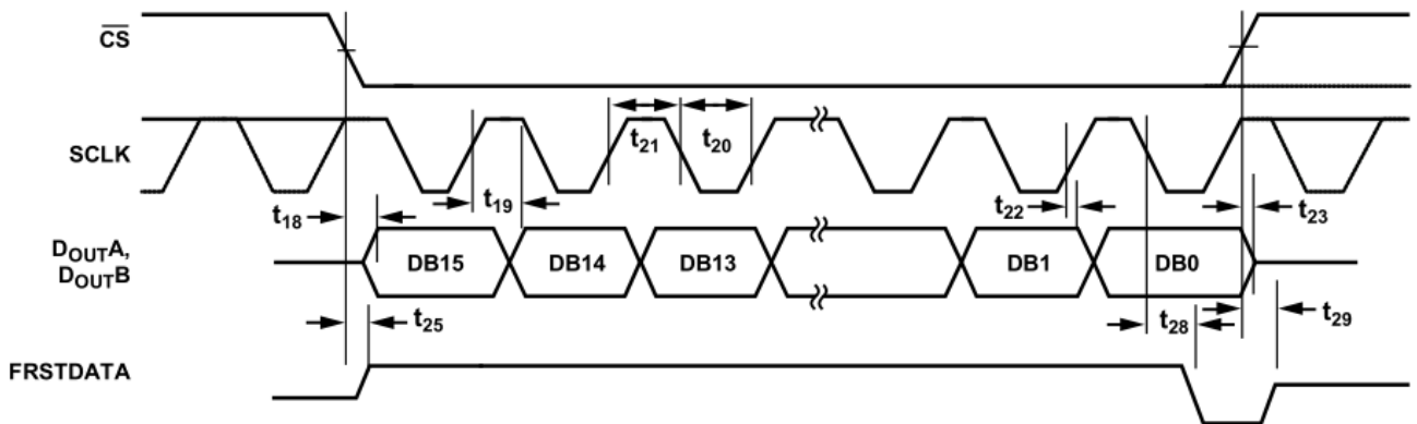
图 7 串行接口模式 (通道 1)
