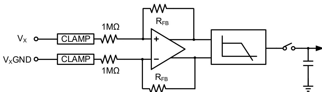
图 10 模拟输入电路
