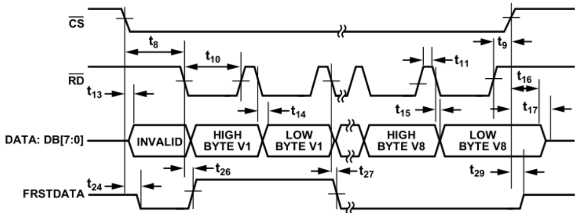
图 8 并行字节接口模式
