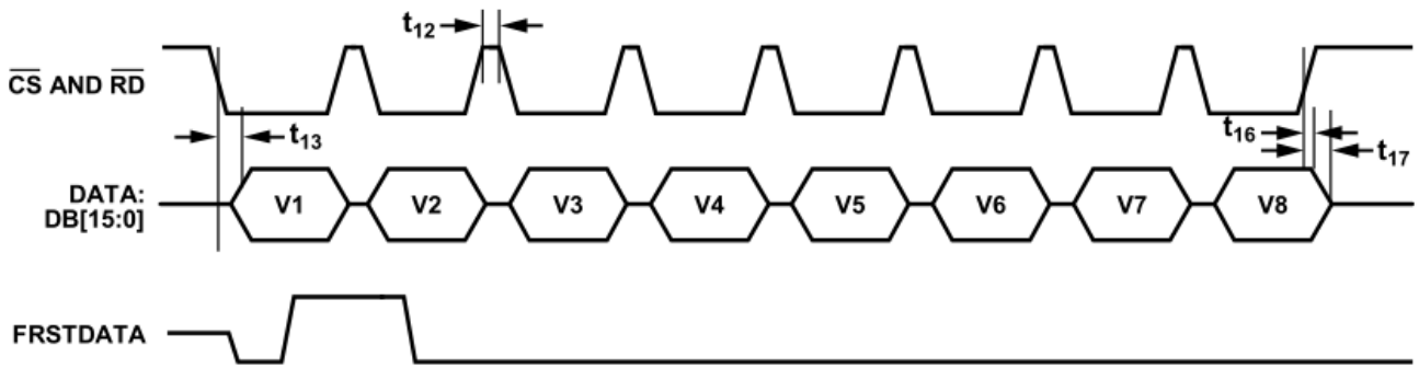
图 6 并行接口模式 (CS 和 RD 相连)
