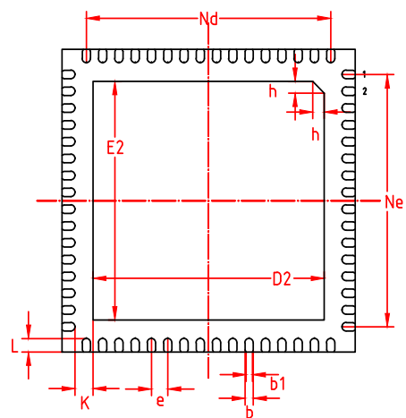
机械尺寸/mm
