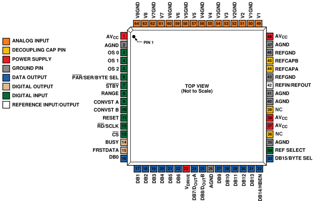
图 2 HT7606 引脚配置图
