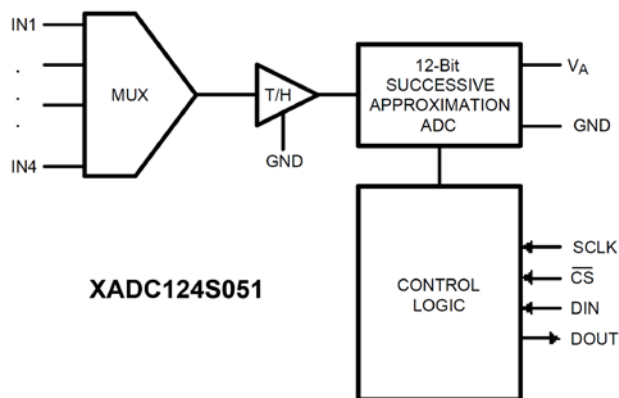
原理图
