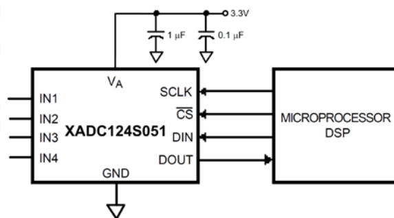
典型连接电路图
