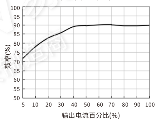
效率Vs输出负载(Vin=48V) URA4815LD-20WR3
