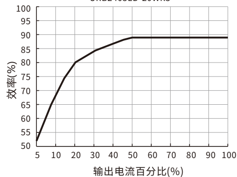
效率Vs输出负载(Vin=24V) URB2405LD-20WR3
