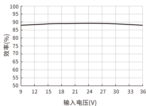
效率Vs输入电压(满载) URB2405LD-20WR3
