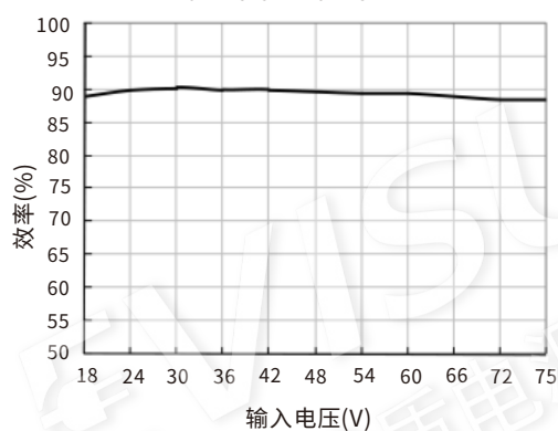
效率Vs输入电压(满载) URA4815LD-20WR3
