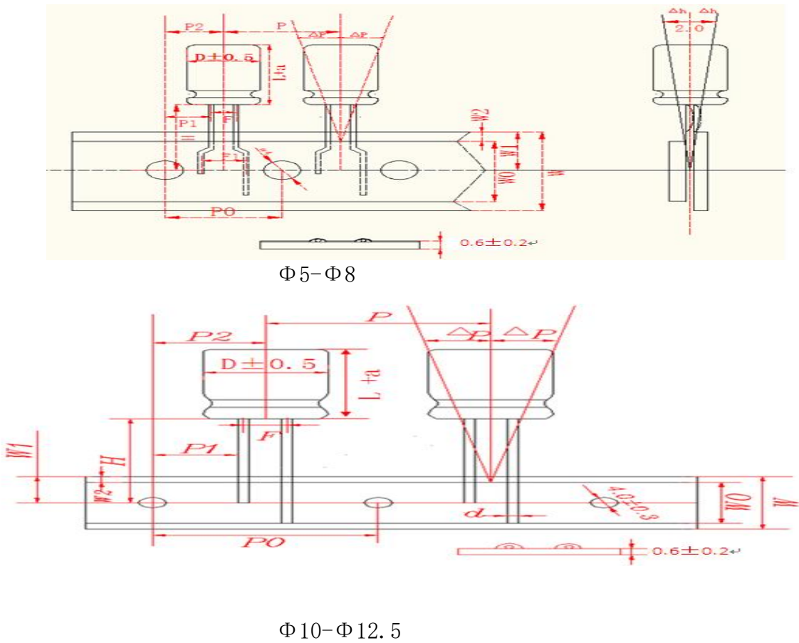
编带外型尺寸 B 图
