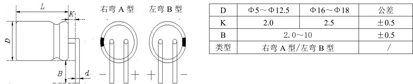
引线切脚成型 F 图（成型折弯 90°）
