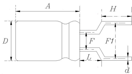
引线切脚成型 G 图
