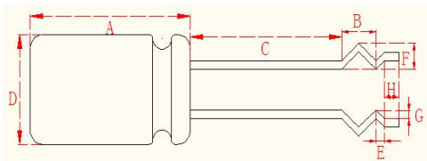
引线切脚成型 C 图
