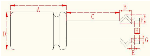
引线切脚成型 C 图
