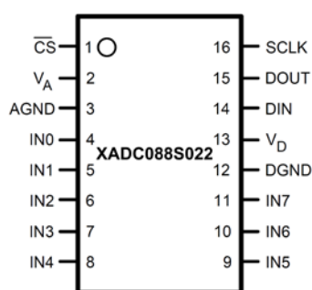
引脚图
