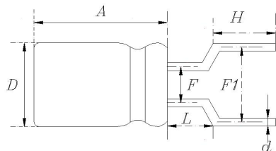
引线切脚成型 G 图
