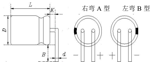
引线切脚成型 F 图 （成型折弯 90°）
