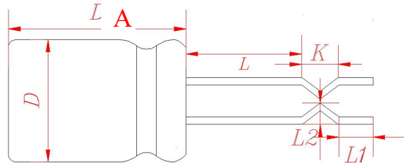
引线切脚成型 E 图
