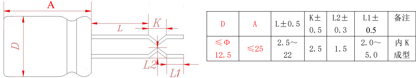
引线切脚成型 E 图
